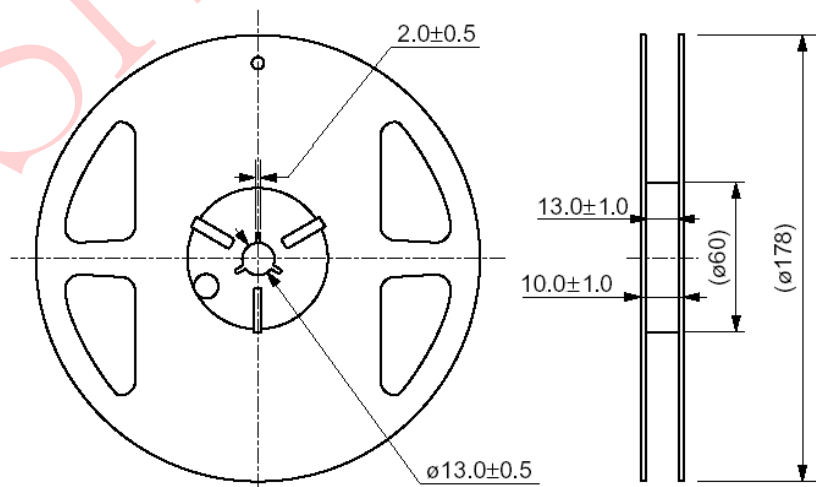
⌀178 Reel Dimension
